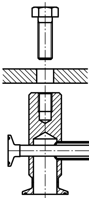
MONTÁŽNÍ OTVOR SE ZÁVITEM
