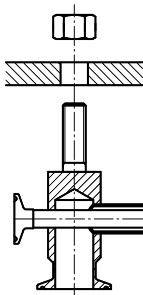
MONTÁŽNÍ ČEP SE ZÁVITEM
